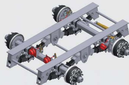
Pevný nebo natáčecí snížený tandem
